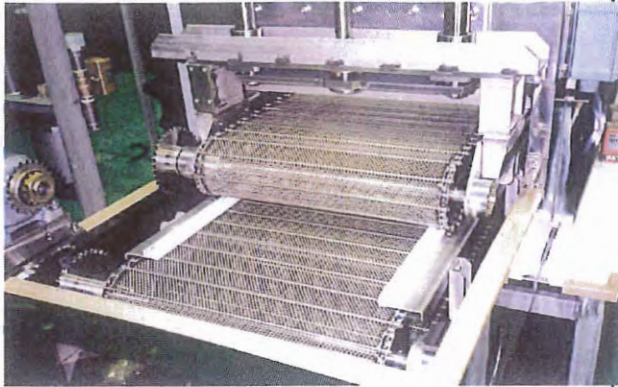
ネットコンベアー式洗浄機
