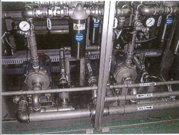
配管部
