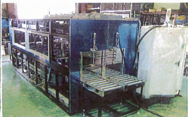
水溶性4槽プッシャー式洗浄機
